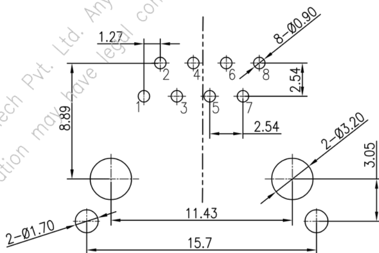
P.C.B LAYOUT
