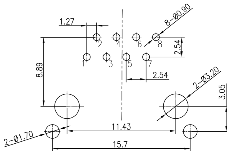
P.C.B. LAYOUT
