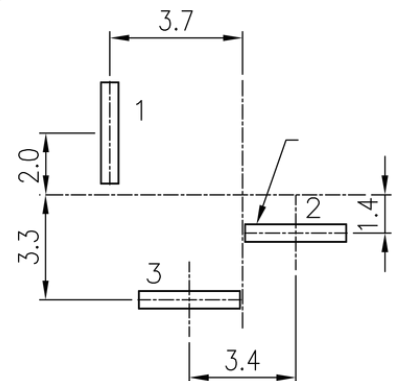
P.C.B LAYOUT
