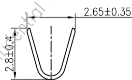
SEC-AA
