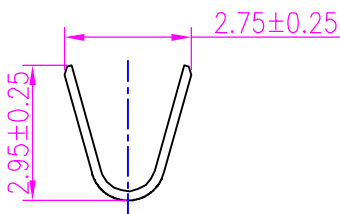
SEC-AA
