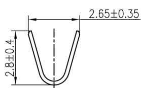
SEC-AA
